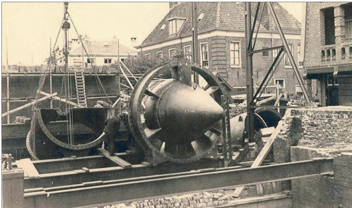
Bouw van het gemaal met schroefpomp.
