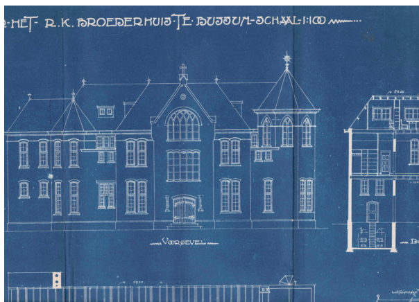
Bouwtekening van het Broederhuis aan de St.-Vitusstraat
