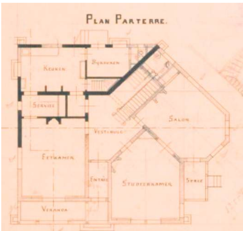
■ Bouwtekening van de begane grond van Villa Tsjido.
